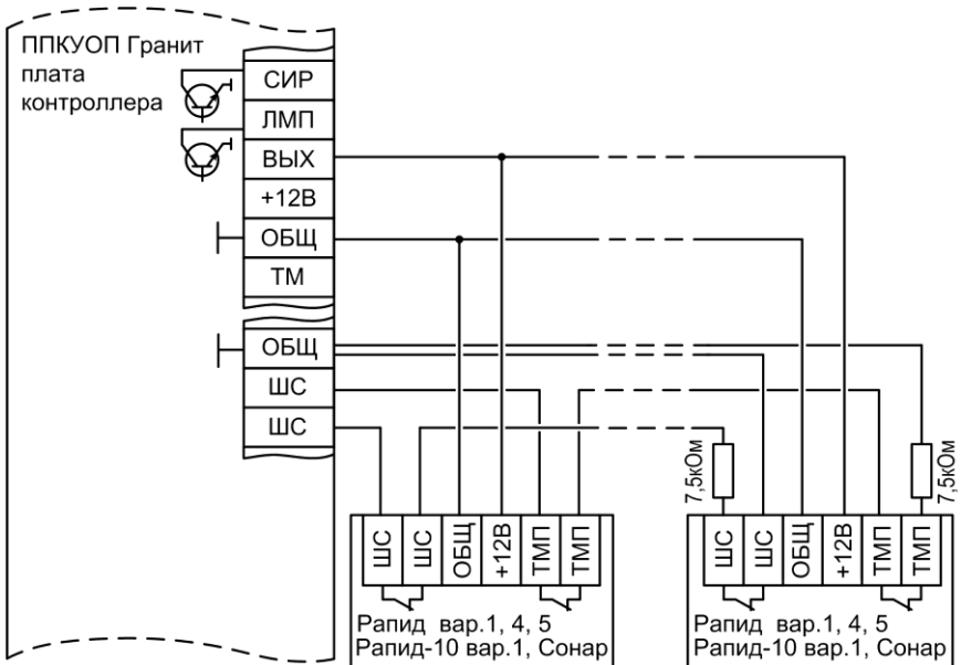
Рис.А3 Схема подключения охранных извещателей Rapid вар.1,4,5, Rapид-10 вар.1, Сонар (тампер извещателя подключён к отдельному ШС)
