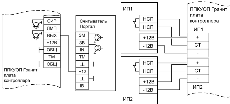
Рис.А5 Схема подключения считывателя «Портал»
